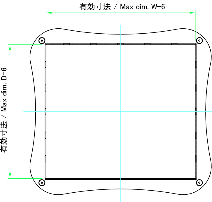
下カバー / Bottom cover
